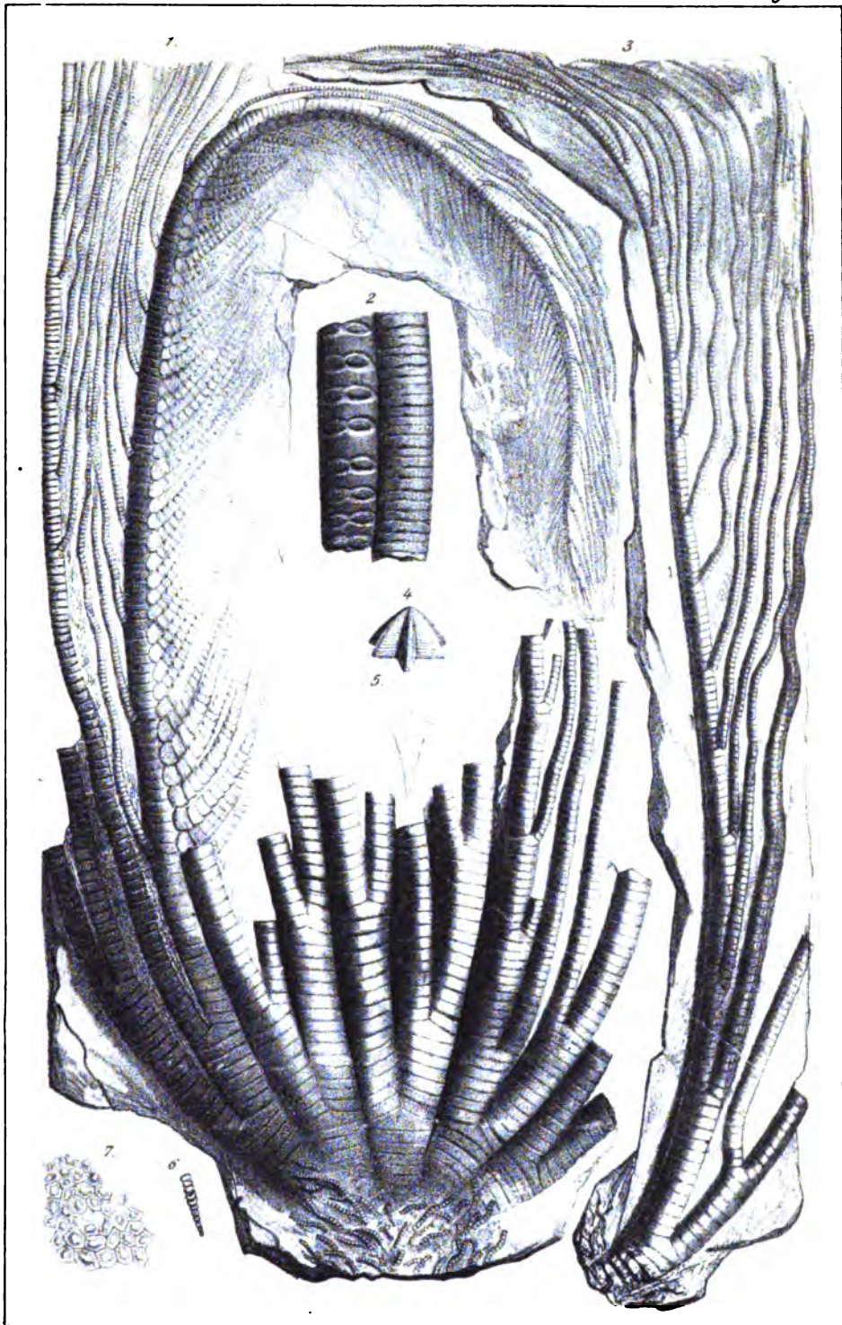
Quenstedt, Jura.
